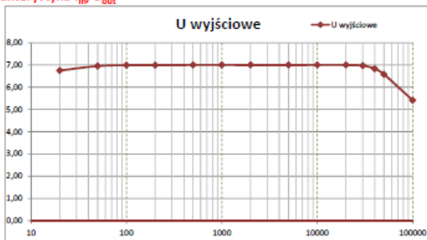
Charakterystyka f_{in}/U_{out}
